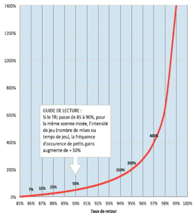
Figure 1: Taux de retour au joueur et fréquence d'occurrence des gains
